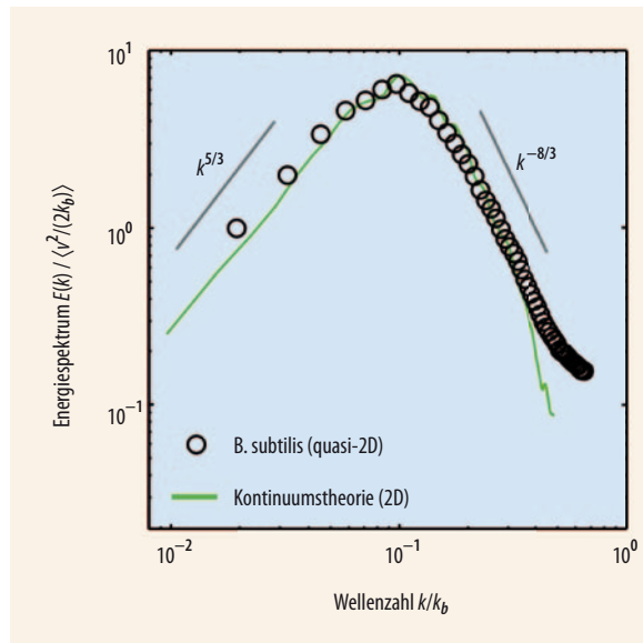
Abb. 1 Das Energiespektrum zweidimensionaler bakterieller Suspensionen folgt bei großen und kleinen Wellenzahlen Potenzgesetzen. Kontinuumstheorie und Experiment stimmen sehr gut überein. Das deutet auf einen neuen universellen Mechanismus der „aktiven Turbulenz“ hin. Hierbei bezeichnen \langle v^2/2 \rangle die mittlere kinetische Energie und k_b die Wellenzahl, die der Bacillus-Länge entspricht.
